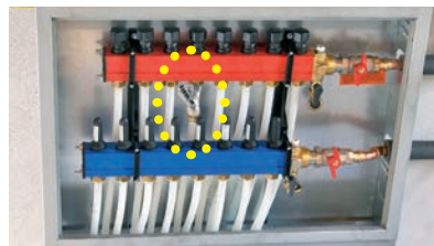
Einbau im Fußboden-Heizkreisverteiler
