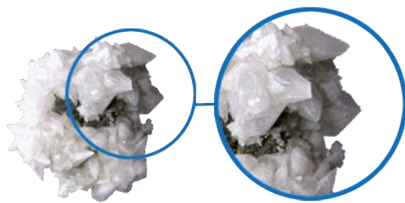
Calcit (vorher)
